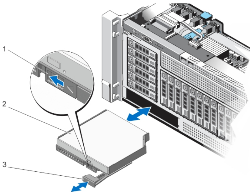
Abbildung 25. Entfernen und Installieren des optischen Laufwerks
