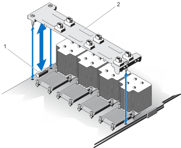
Abbildung 27. Entfernen und Installieren des Lüfterauflagefachs
