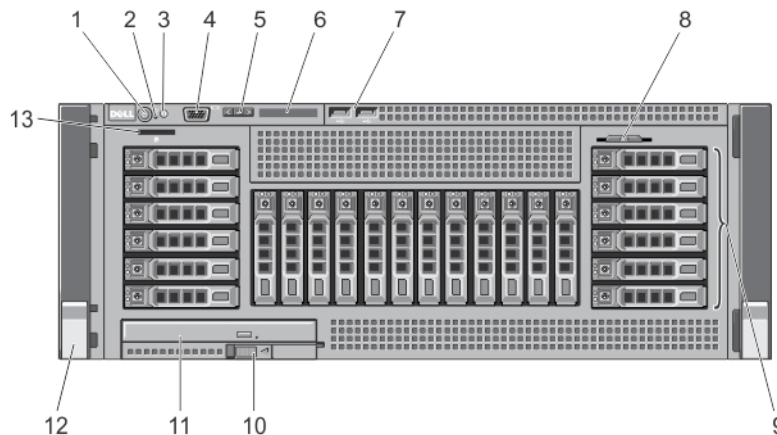
Abbildung 1. Merkmale und Anzeigen auf der Vorderseite
